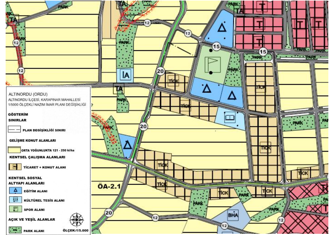
Öneri Plan
